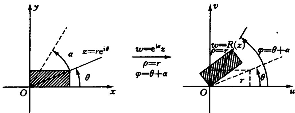
图 6-7 旋转映射 w = e^{i\alpha} z
