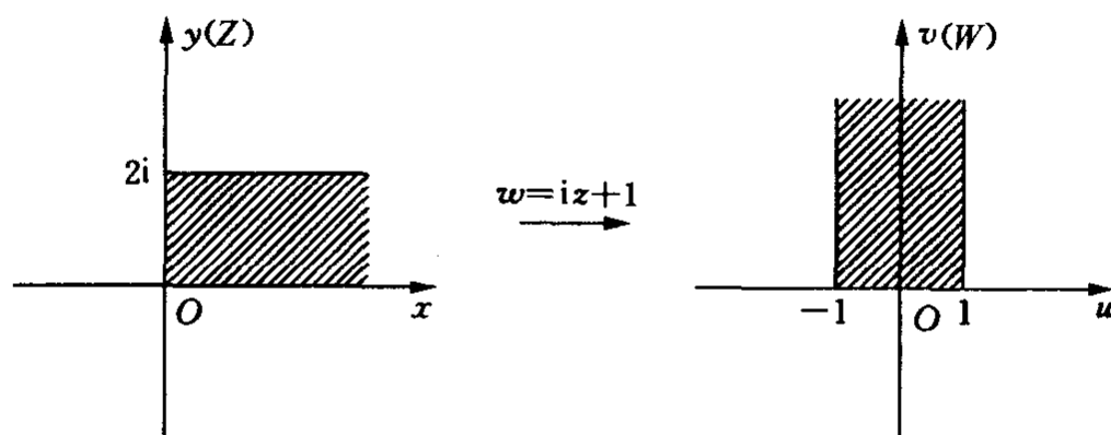
图 6-32 w = iz + 1
