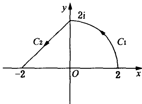
图 3-2 C_1 与 C_2
