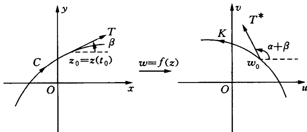
图 6-1 过 z_0 点曲线 C 的切向量 T 与过 w_0 点曲线 K 的切向量 T^* , f'(z_0) \neq 0
