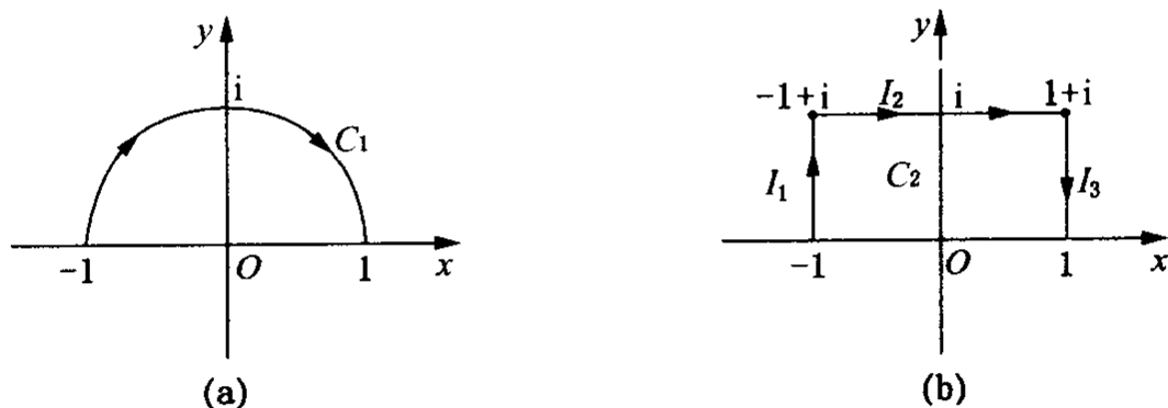
图 3-6 C_1 与 C_2
