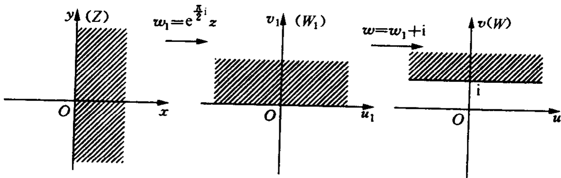
图 6-30 w = iz + i
