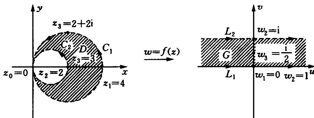
图 6-18 映射 w = -i \frac{z-4}{z}
