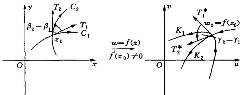
图 6-2 f'(z_0) \neq 0 时, 解析函数 w = f(z) 在 z_0 点是保角的, \gamma_2 - \gamma_1 = \beta_2 - \beta_1
