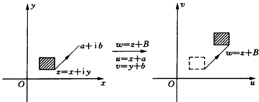
图 6-6 平移映射 w = T(z) = z + B
