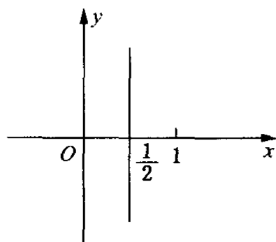
图 1-12 \{z; |z-1|=|z|\}
