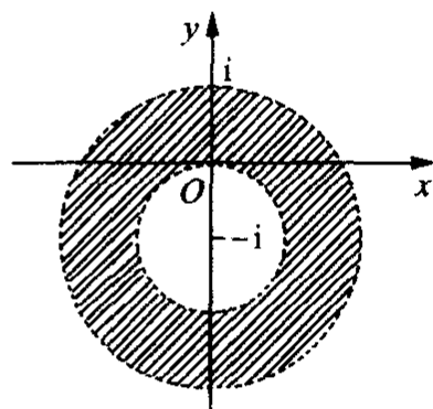
图 1-14 \{1 < |z+i| < 2\}
