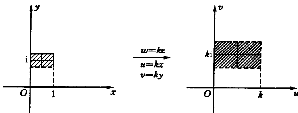
图 6-8 伸缩映射 w = kz
