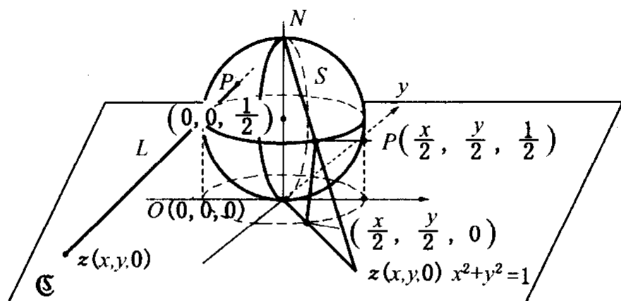
图 1-1 复球面
