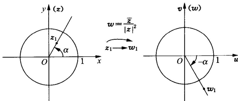
图 1-9 倒置映射
