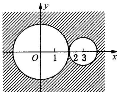
图 1-15 \{z; \operatorname{Im} z > 1 \text{ 且 } |z| < 2\} 图 1-16 \{z; |z| > 2 \text{ 且 } |z-3| > 1\}
