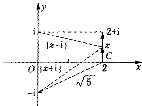
图 3-3 |z-i| 与 |z+i|
