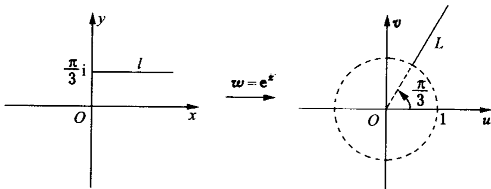
图 2-1 映射 w = e^z 将 l 映射到 L
