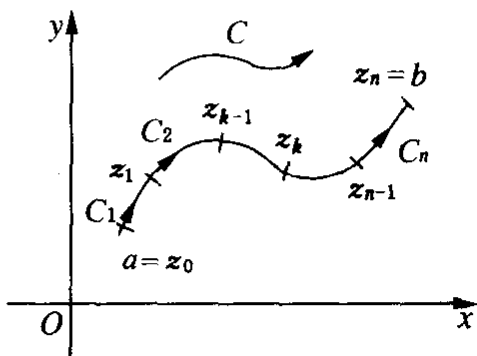
图 3-1 有向曲线 C 的分割
