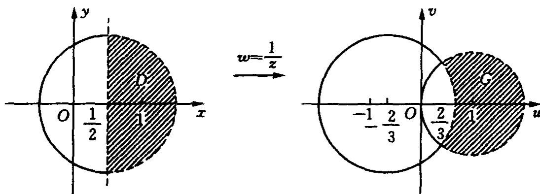
图 6-11 w = \frac{1}{z} 将 D 映射为 G
