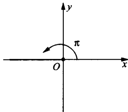
图 1-11 \{z; \arg z = \pi\}
