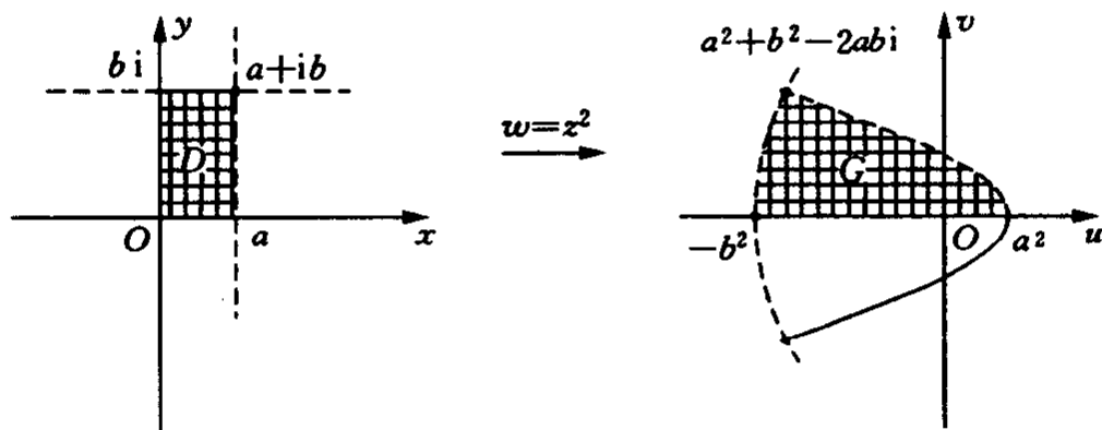
图 6-14 映射 w = z^2 将区域 D 映射成区域 G
