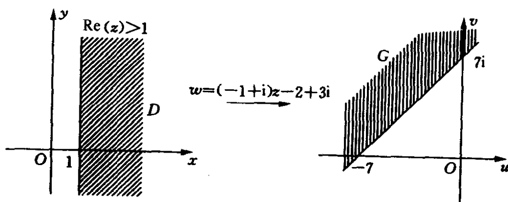
图 6-9 映射 w = (-1 + i)z - 2 + 3i
